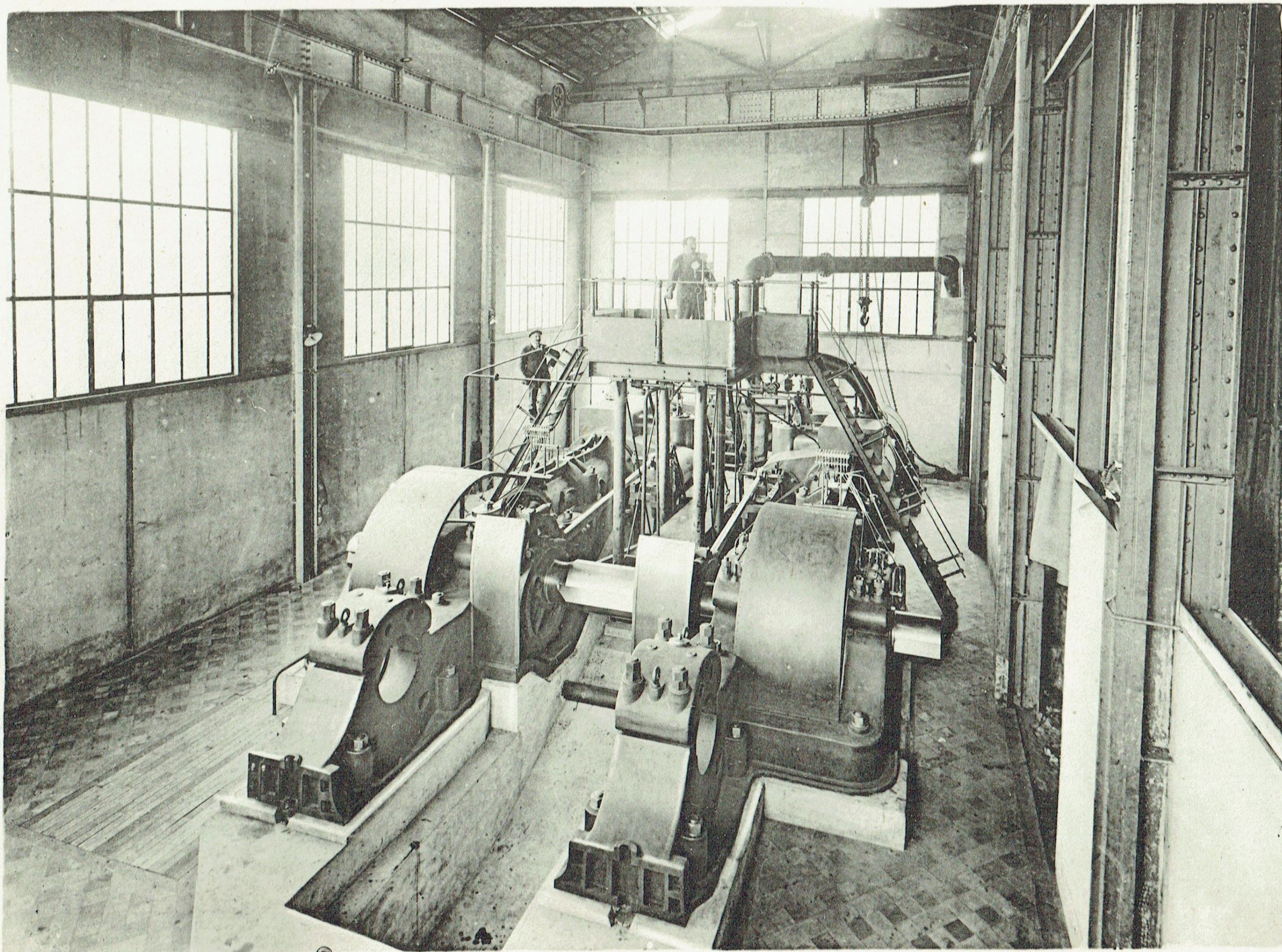
Marnaval - Machine réversible du blooming
