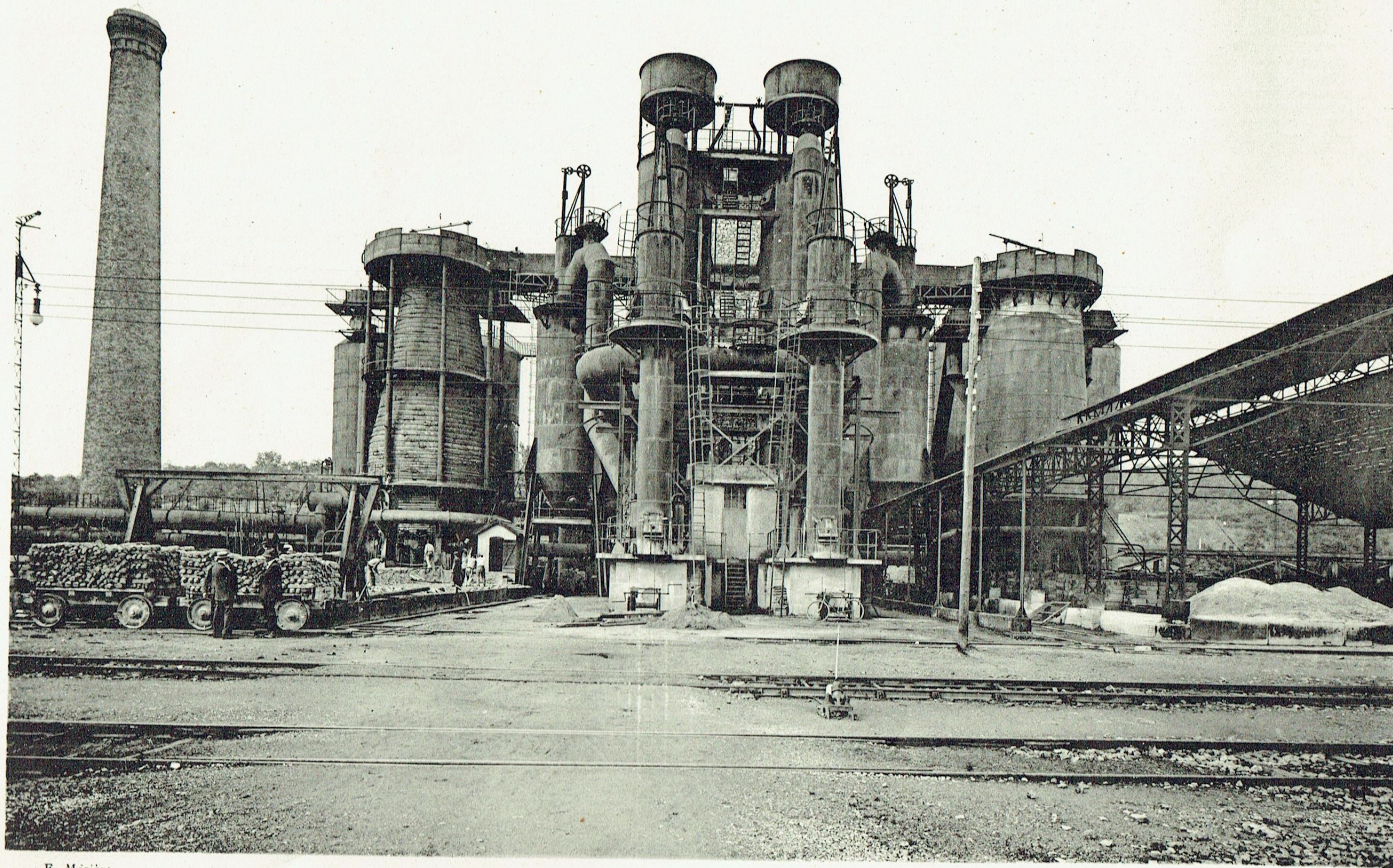
Marnaval - Hauts-fourneaux 1 et 2
