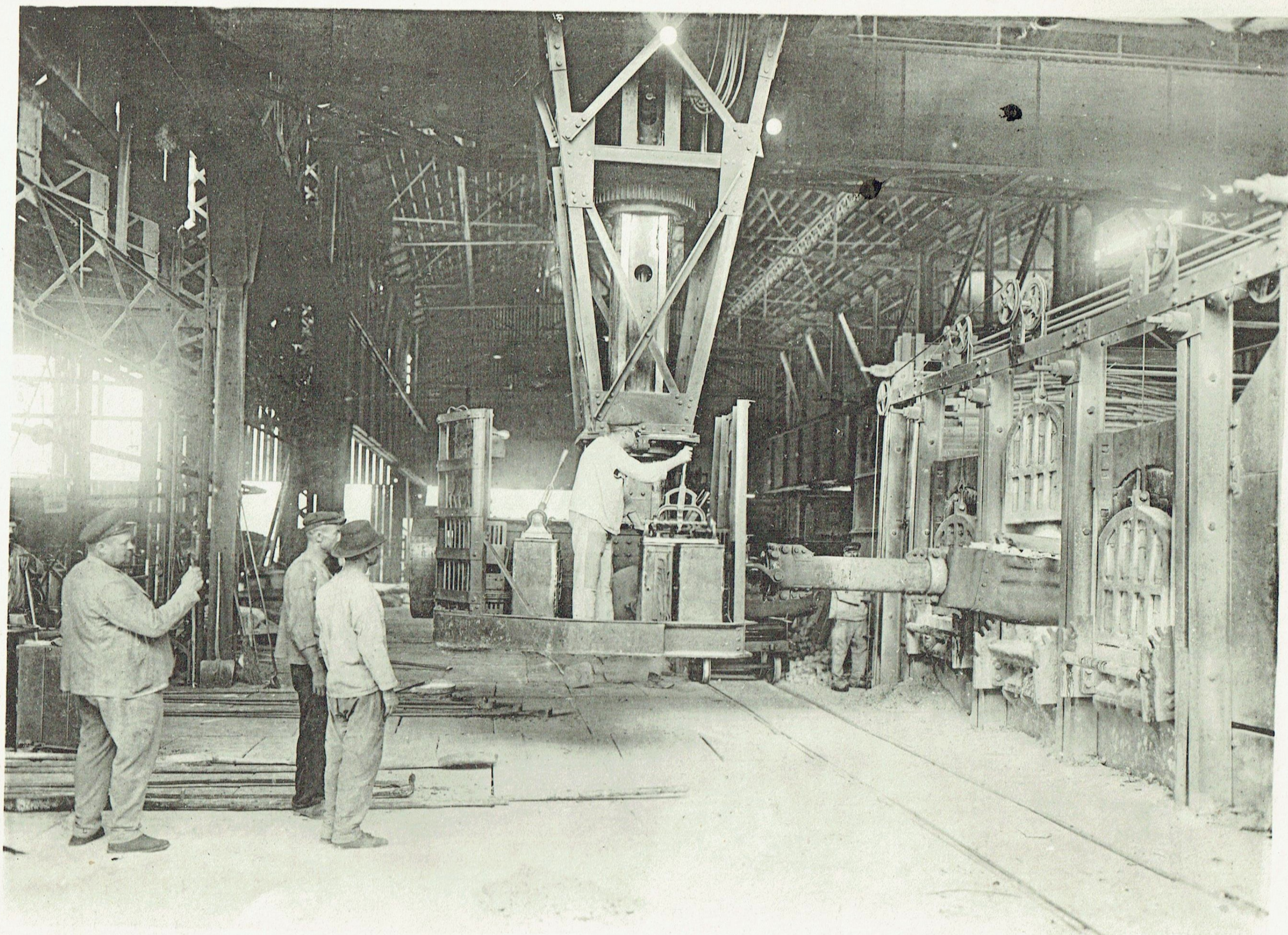
Marnaval - Chargement d'un four Martin
