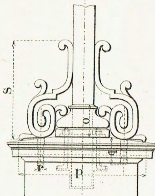
Embase à consoles
