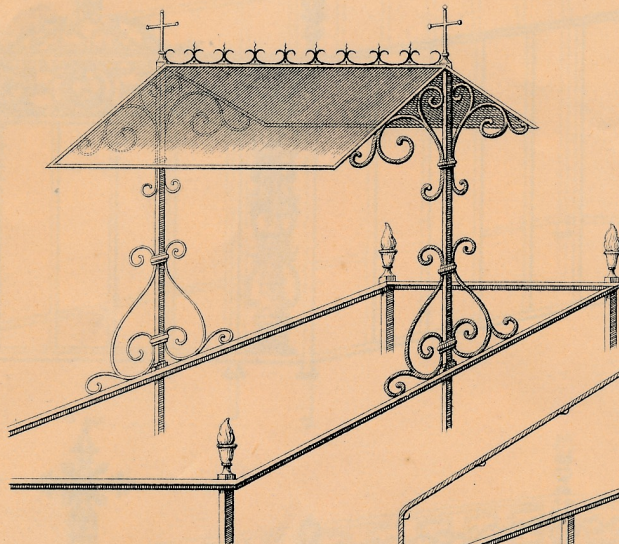
Couvre-couronnes N° 2
